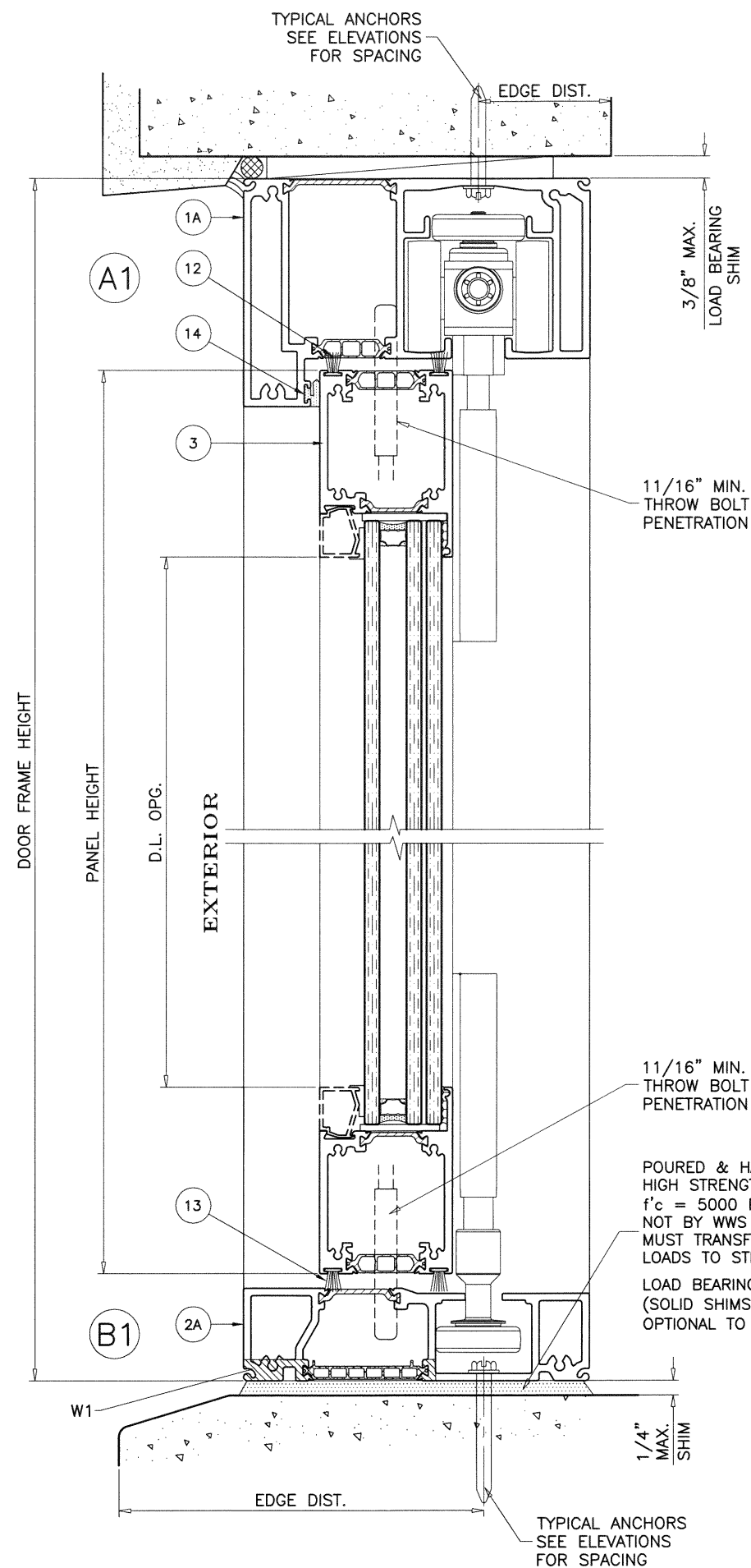
E-4 FRAME OPTION
